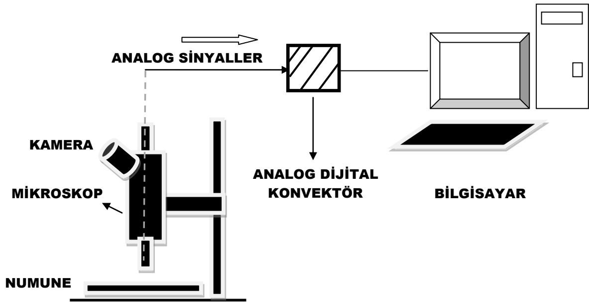
Şekil 1. Görüntü Analiz Cihazı şematik gösterimi
